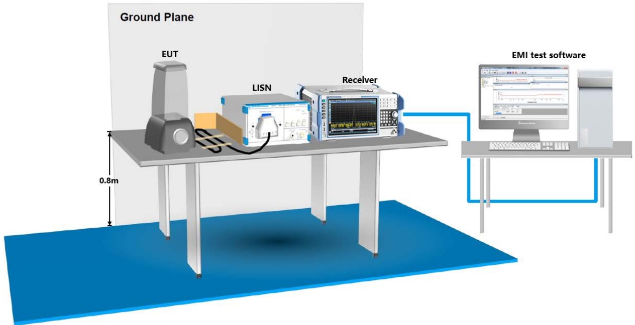
图一：EMI-CE300 进阶版 EMI 诊断测试系统示例
