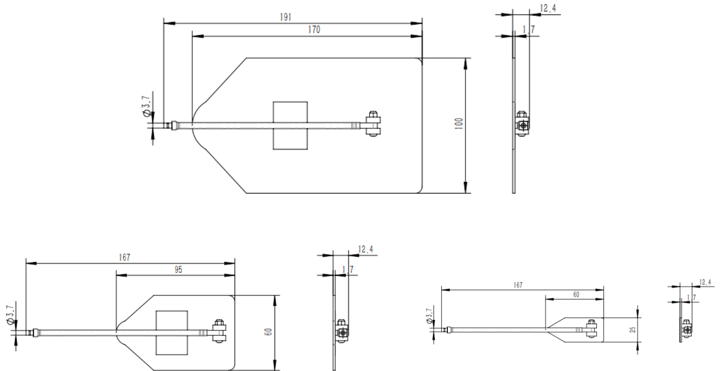
尺寸图
